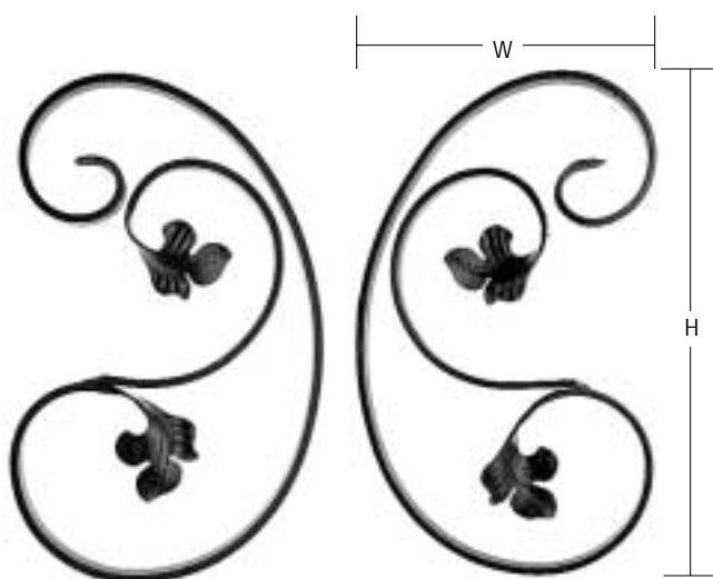
BS-635 — 1/4" x 1/2" 9"W x 15"H
