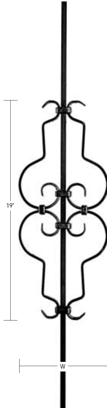
P-1393 ■ 1/2" 10"W x 39"H
